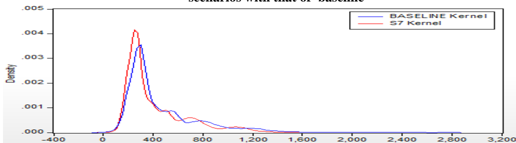
نمودار (۱۰) مقایسه نمودار توابع چگالی احتمال ترکیبی عملکرد گندم دیم بر مبنای سناریو هفتم با حالت پایه
