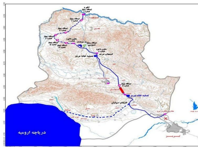
شکل (۱) مسیر انتقال آب از رود ارس به دریاچه ارومیه
