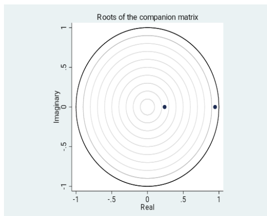
شکل (۱) ریشه‌های ماتریس و شرط پایداری
