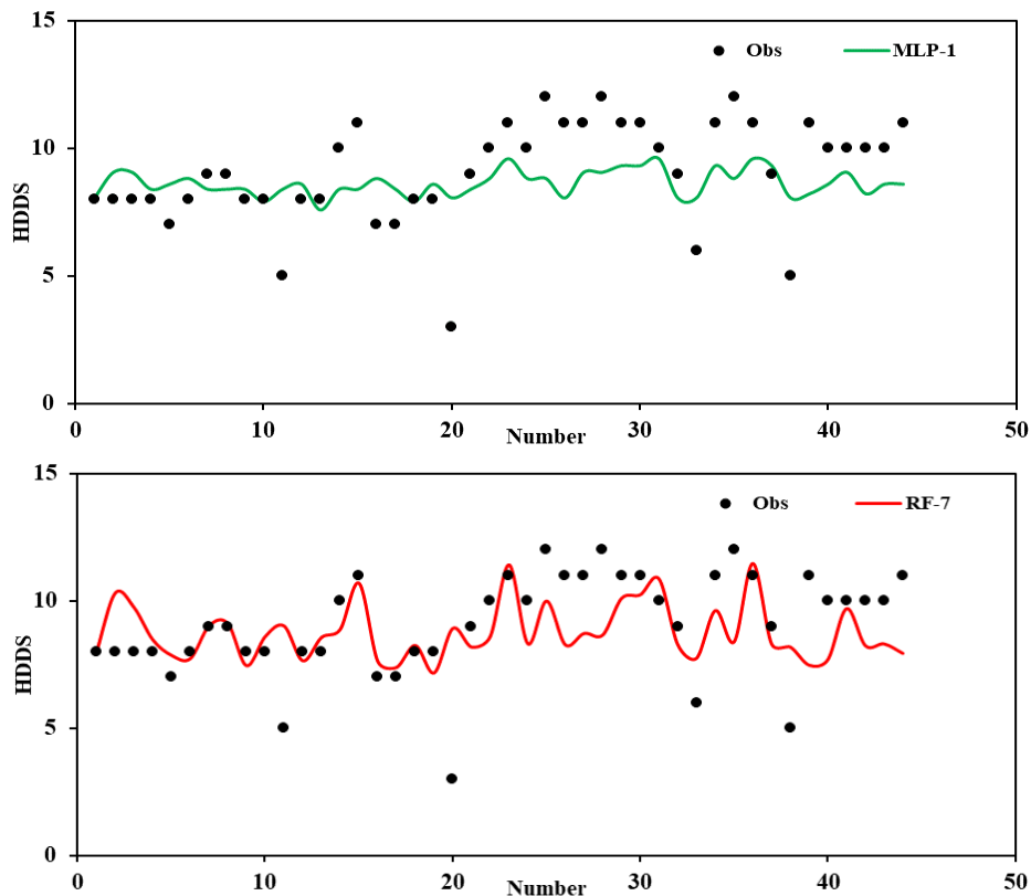
شکل (۳) اختلاف HDDS مشاهده شدنی و پیش‌بینی شده با استفاده از مدل‌های MLP-1 و RF-7 Figure (3) Difference of observed and predicted HDDS using MLP-1 and RF-7 models
