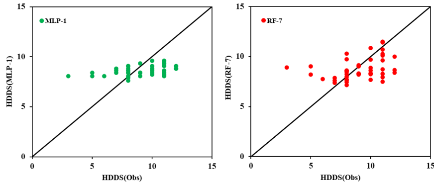
شکل (۵) نمودارهای پراکنش HDDS مشاهده شدنی و پیش‌بینی شده با استفاده از مدل‌های MLP-1 و RF-7 Figure (5) Scatter plots of observed and predicted HDDS using MLP-1 and RF-7 models
