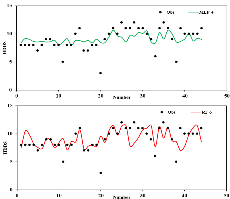
شکل (۲) اختلاف مشاهده‌شده و پیش‌بینی شده با استفاده از مدل‌های MLP-4 و RF-6 Figure (2) Difference of observed and predicted HDDS using MLP-4 and RF-6 models
